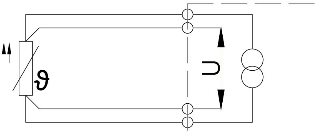
Vierleiter four-wire
